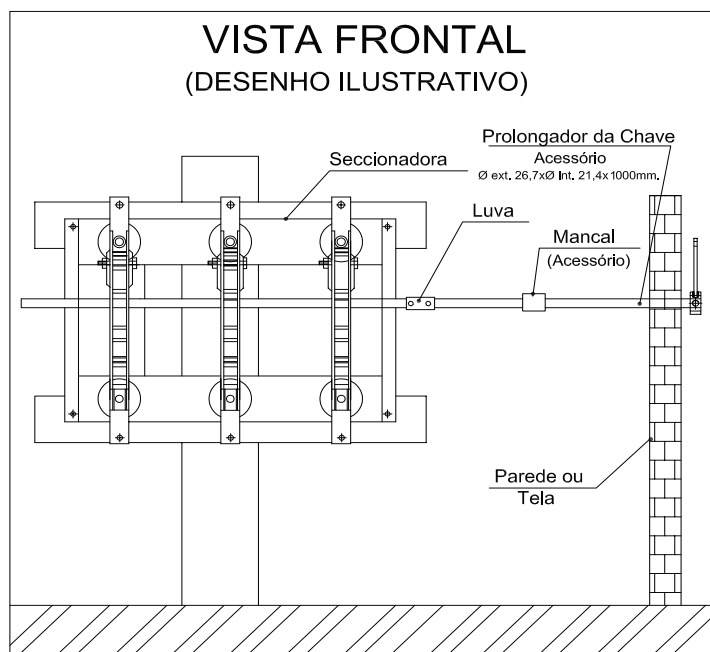
Figura 03 – Instalação da chave com prolongador da chave.
