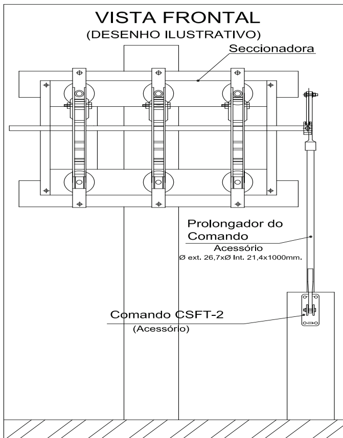
Figura 02 – Instalação da chave com prolongador do comando.
