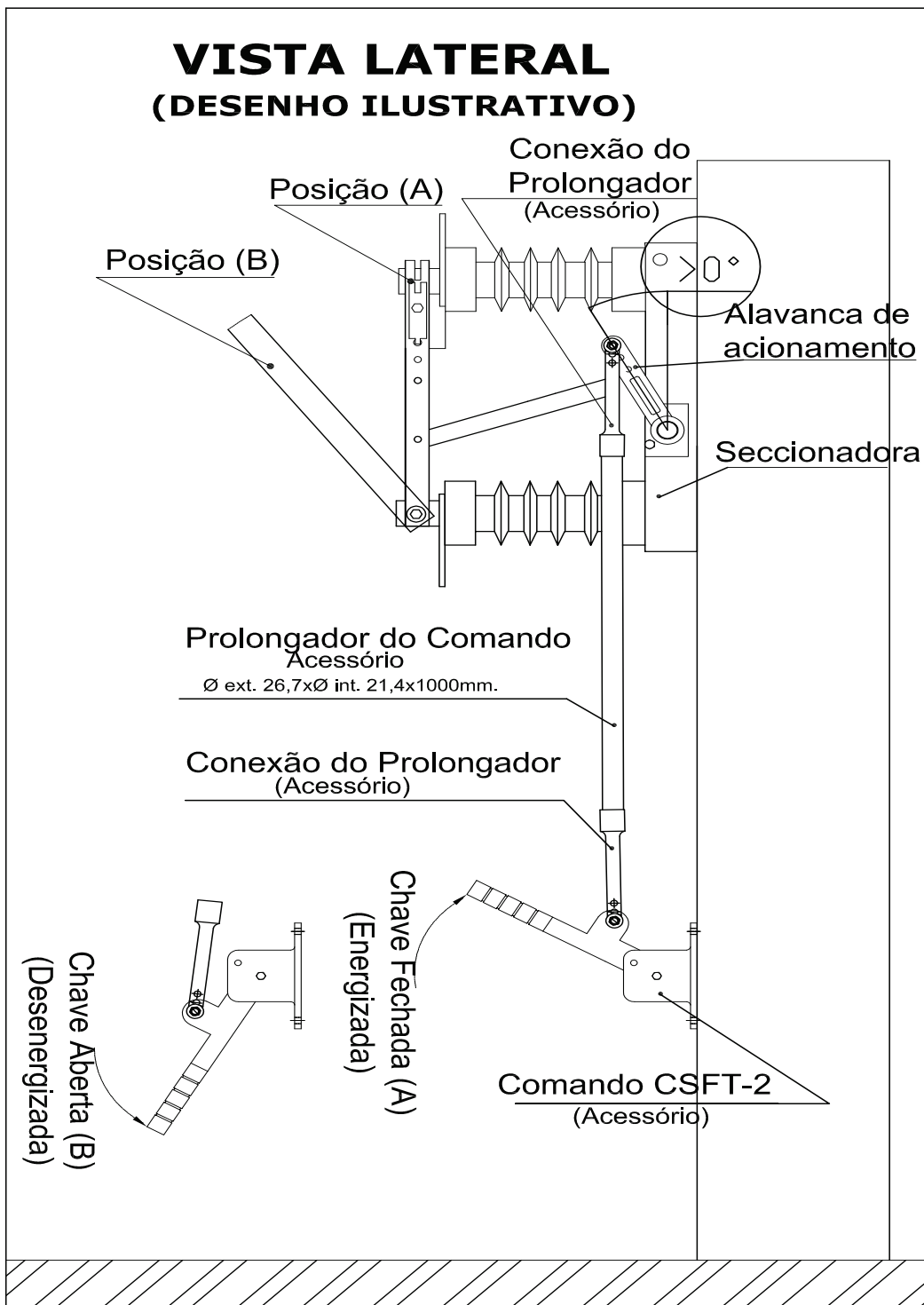
Figura 04 – Instalação da chave com prolongador do comando e com ou sem prolongador da chave
